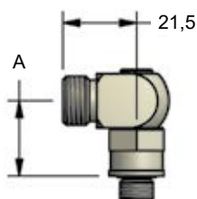
90.506.230 (S-230) 90° Obracać
