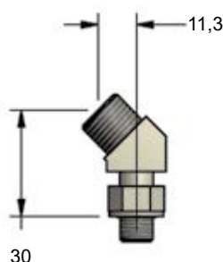
90.505.330 (S-330) 45° Obracać
