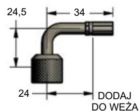
90.804.959 Długo 90° Adapter Węży (B-959)
