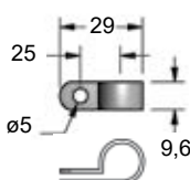
90.504.250 (HS-250) do użytku z wężami typu 90.500, 90.400 i 90.250
