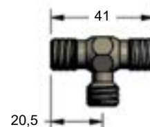
90.806.401 Trójnik
