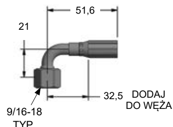
90.504.559 (SK-559) 90° Obracać
