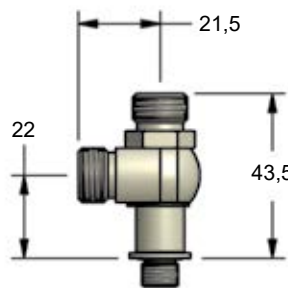
90.505.438 (S-438) Trójkąt Obracać
