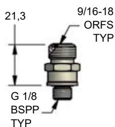
90.505.115 (S-115) Prosto
