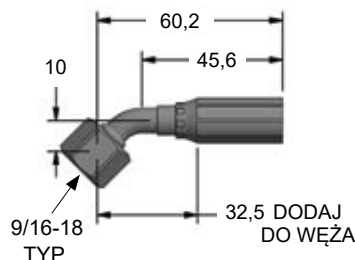
90.504.454 (SK-454) 45° Obracać
