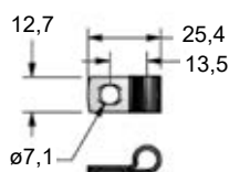
90.504.700 (HS-700) do użytku z 90.700 i 90.705 typów węży
