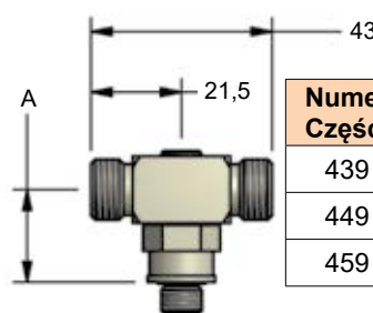
90.506.439 (S-439) Trójkąt Obracać
