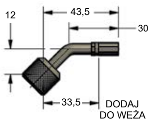
90.804.954 45° Adapter Węży (B-954)
