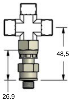
90.505.121 (S-121) Obracać Prosto
