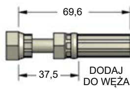
90.504.751 (S-751) Chowany Obracać
