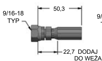
90.504.443 (SK-443) Kompaktowy Obracać
