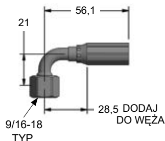
90.504.459 (SK-459) 90° Obracać
