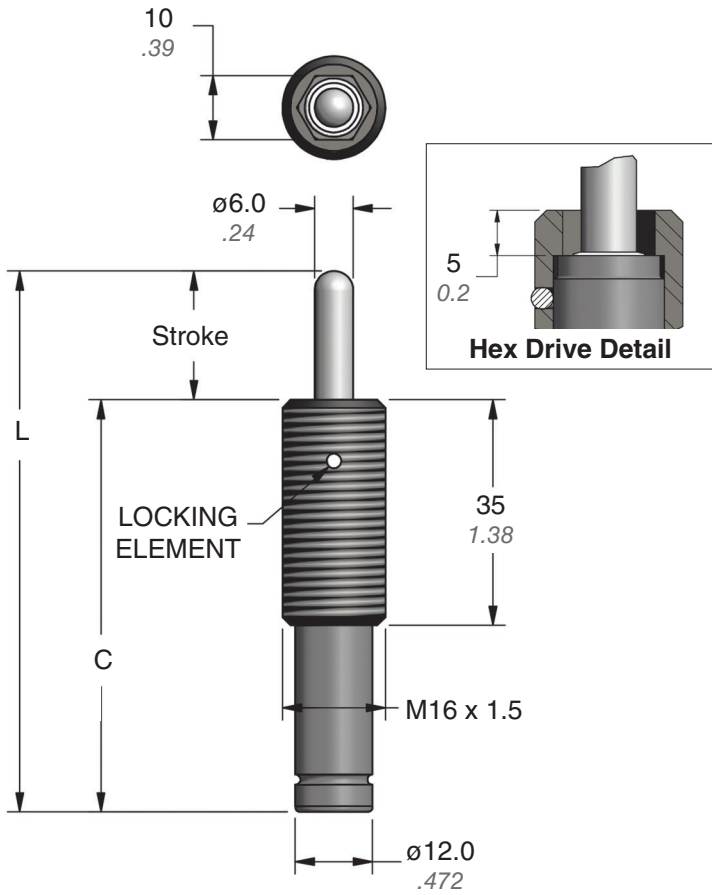
Jam Nut SL-16-JN
