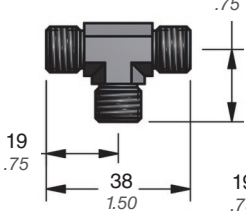
90.508.401 (D-401) Tee
