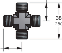
90.508.501 (D-501) Cross
