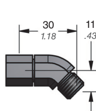
90.508.321 (D-321) 45° Elbow
